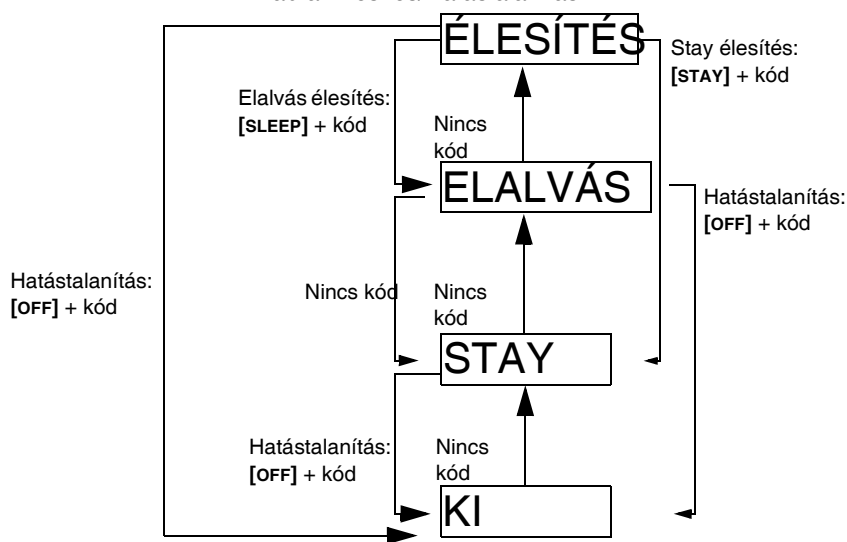
4. ábra: Élesítés/Hatástalanítás
