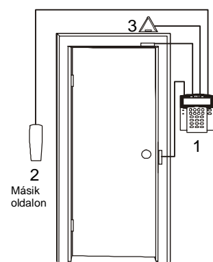
1 = Beléptető LCD Kezelő 2 = Kártyaolvasó 3 = "Kilépés Kérés" Mozgás Érzékelő
