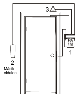
1 = Beléptető LCD Kezelő 2 = Kártyaolvasó 3 = "Kilépés Kérés" Mozcás Érzékelő
